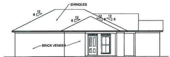
LEFT SIDE ELEVATION SCALE: 1/8" = 1'-0"
