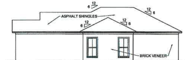
RIGHT SIDE ELEVATION SCALE: 1/8" = 1'-0"
