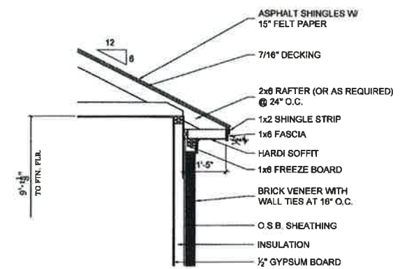
1 TYP WALL SECTION SCALE: 1/2" = 1'-0"
